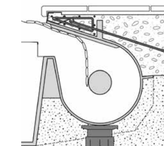
Ausführung bei Becken mit der Bezeichnung „+“
